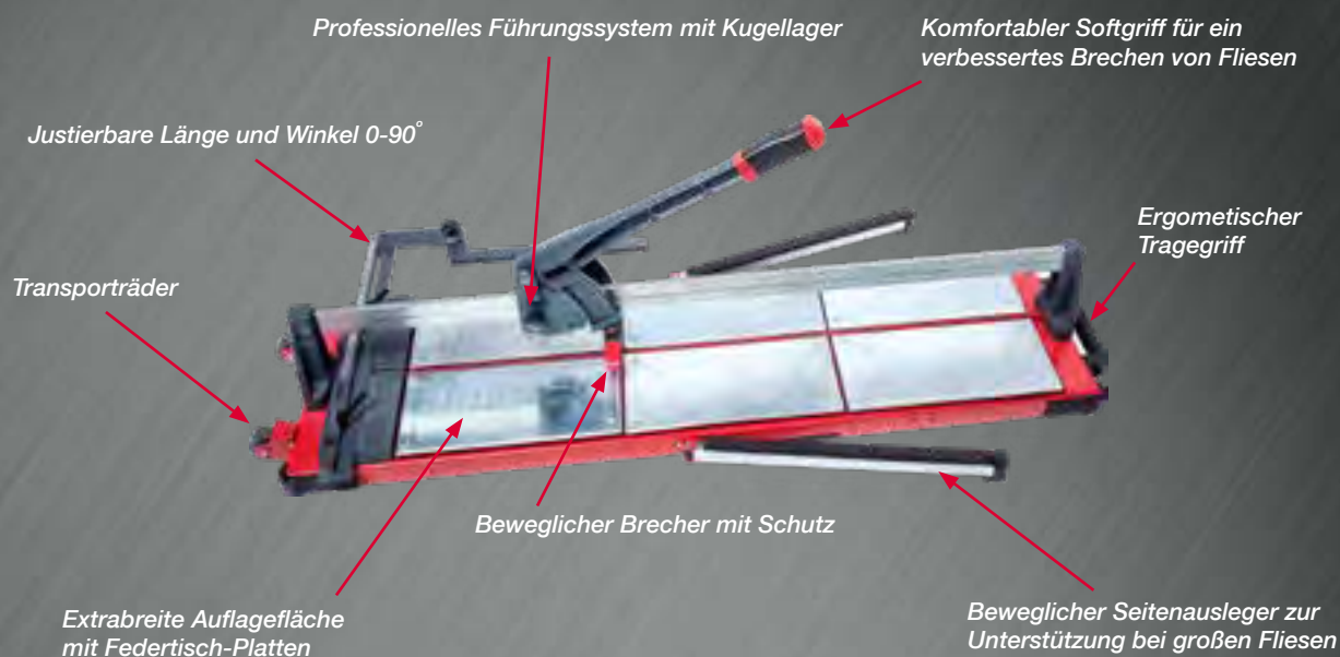
Brechvorrichtung fest justierbar für freis Sicht auf Schneidrad
